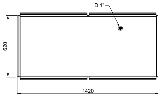
Boven aanzicht
